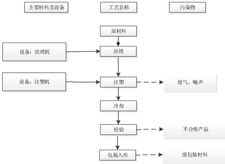
图 2-1 营运期工艺流程及产污位置
