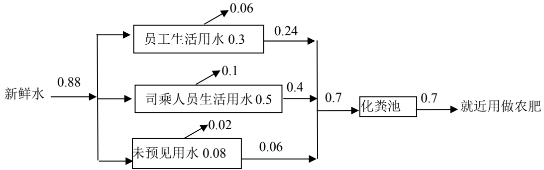
图 1-1 项目水平衡图（消耗单位：m 3 /d）
